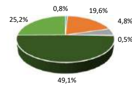
Verbleibender Energieträgermix
